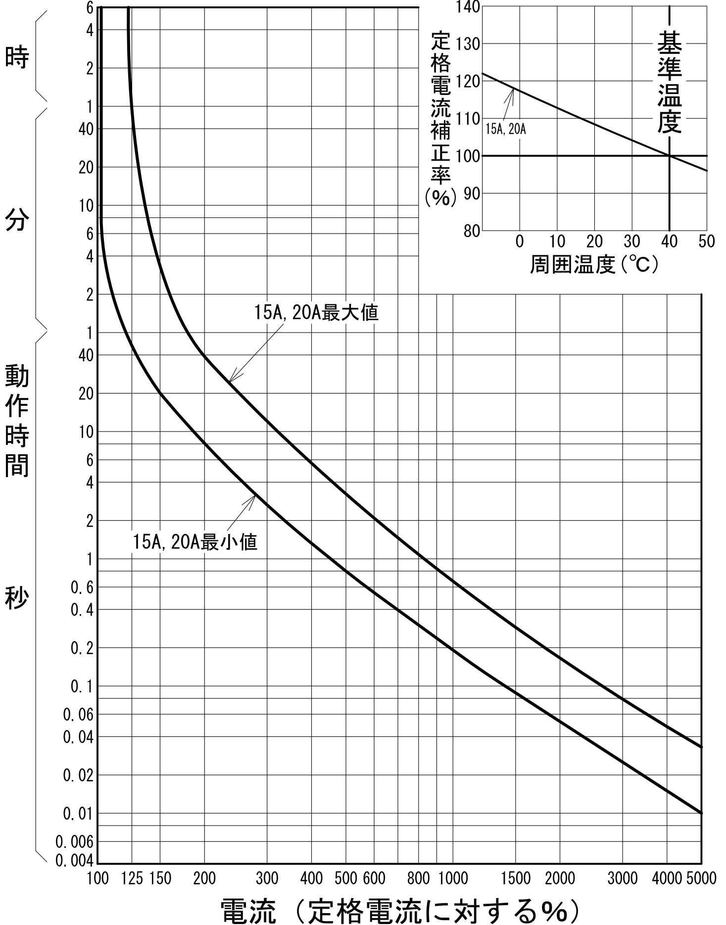
温度補正曲線
