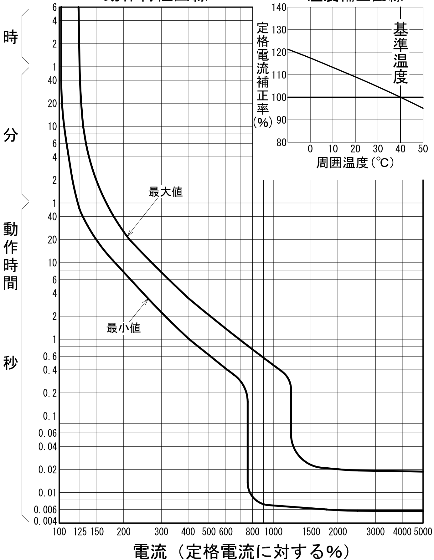
動作特性曲線
